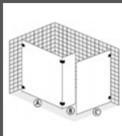
Walk-In Trennwand mit Festfeld/Seitenwand
