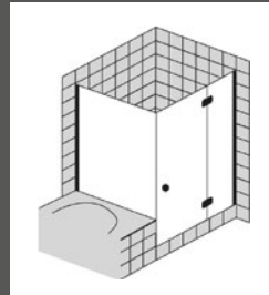
Schwingtür mit Festteil/Seitenwand für Badewanne*
