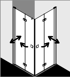
Pendel-Falttür Eckeingangshälfte, 2-tlg.
