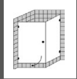
Schwingtür mit Seitenwand
