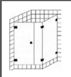
Schwingtür mit Festfeld/ Seitenwand
