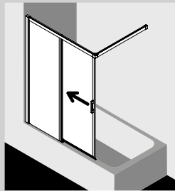
Gleittür 2-tlg. mit Festfeld
