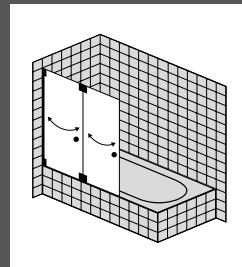
Faltwand 2 tlg. auf Badewanne
