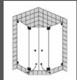
Fünfeckdusche mit 2 Pendeltüren und 2 Festfeldern
