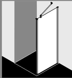
Seitenwand zur Kombination mit Pendeltür oder Pendelfalttür*
